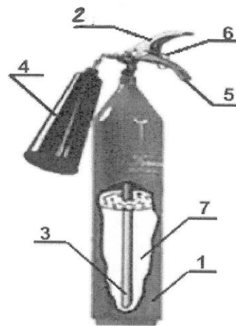
Рисунок А.2 – Устройство переносных углекислотных огнетушителей
