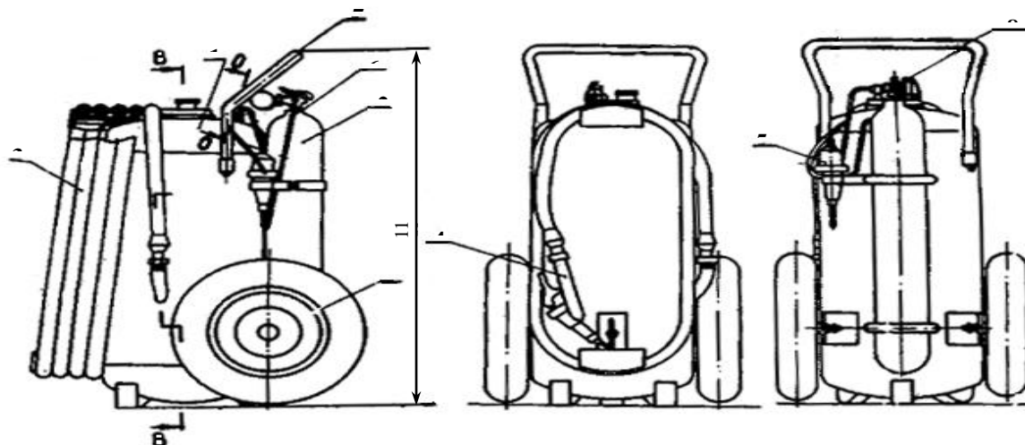
Рисунок А.6 – Устройство огнетушителя ОП-100:
