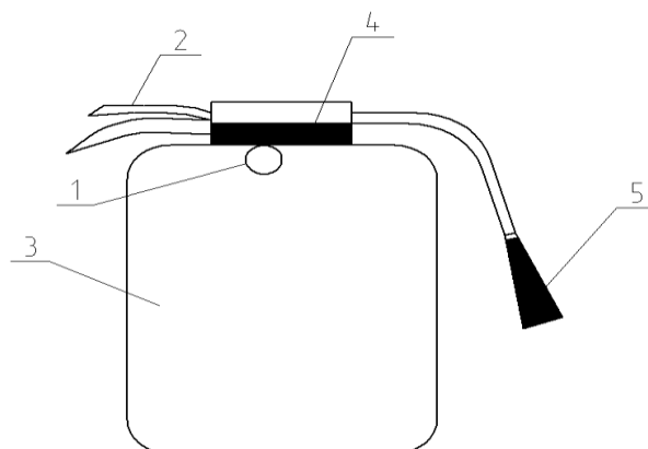
Рисунок А.5 – Устройство огнетушителя порошкового закачного ОП(3):
