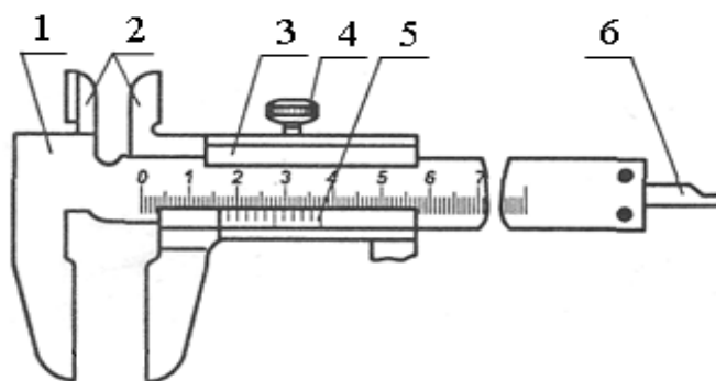
1 – штанга-линейка; 2 – измерительные губки; 3 – рамка; 4 – винт зажима рамки; 5 – нониус; 6 – линейка глубиномера Рисунок 5.1 – Конструкция штангенциркуля типа ШЦ-I
