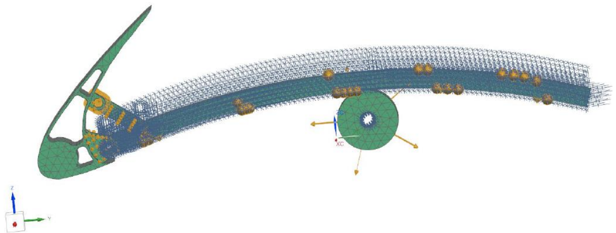
Рисунок 9 – Ограничения
