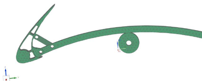
Рисунок 7 – Сеточная модель устройства
