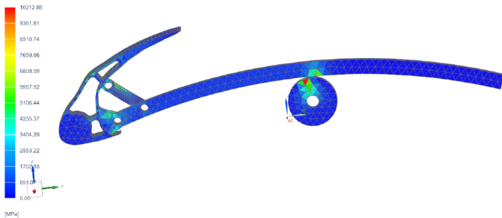
Рисунок 13 – Поле напряжений
