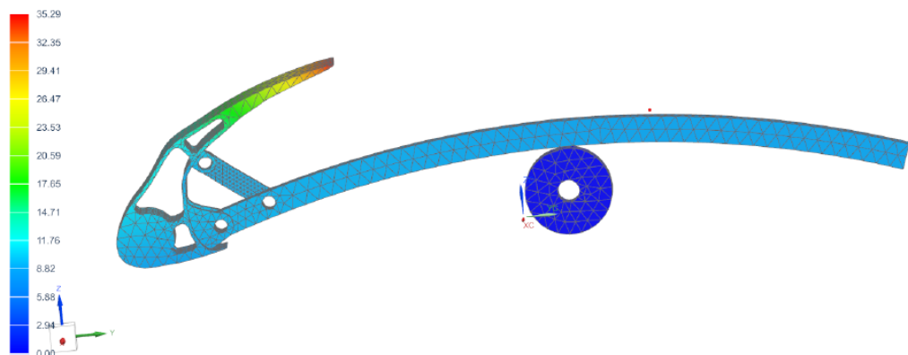
Рисунок 12 – Поле перемещений
