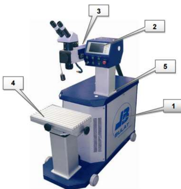
Рисунок 2.3. – Основной блок установки
