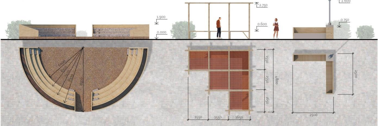
Амфитеатр (1:50)
