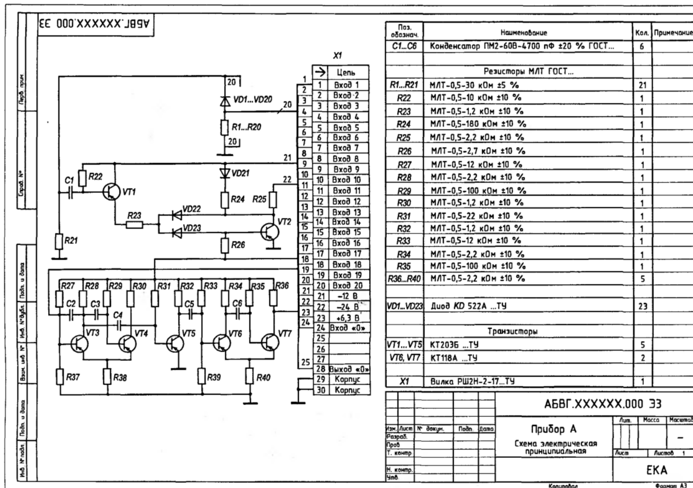
Рис. 6.7. Прибор А. Схема электрическая принципиальная
