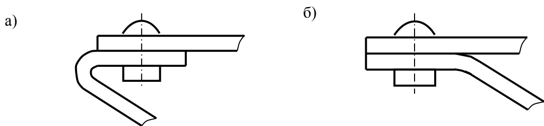
Рисунок 6 – Примеры заклепочных соединений
