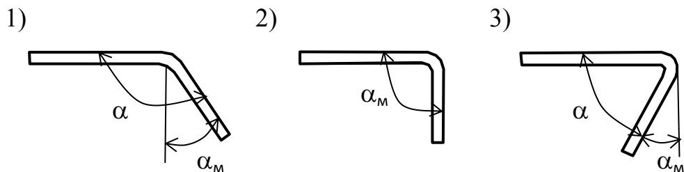
Рисунок 9 – Виды малок
