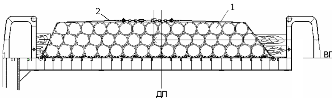
Рисунок 1 – Схема формирования штабеля труб на палубе судна и их крепление: 1- штабель, 2 - найтовы
