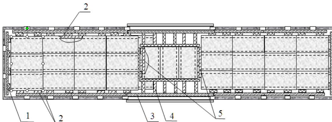
Рисунок 1 - Размещение чушек первичного алюминия:
