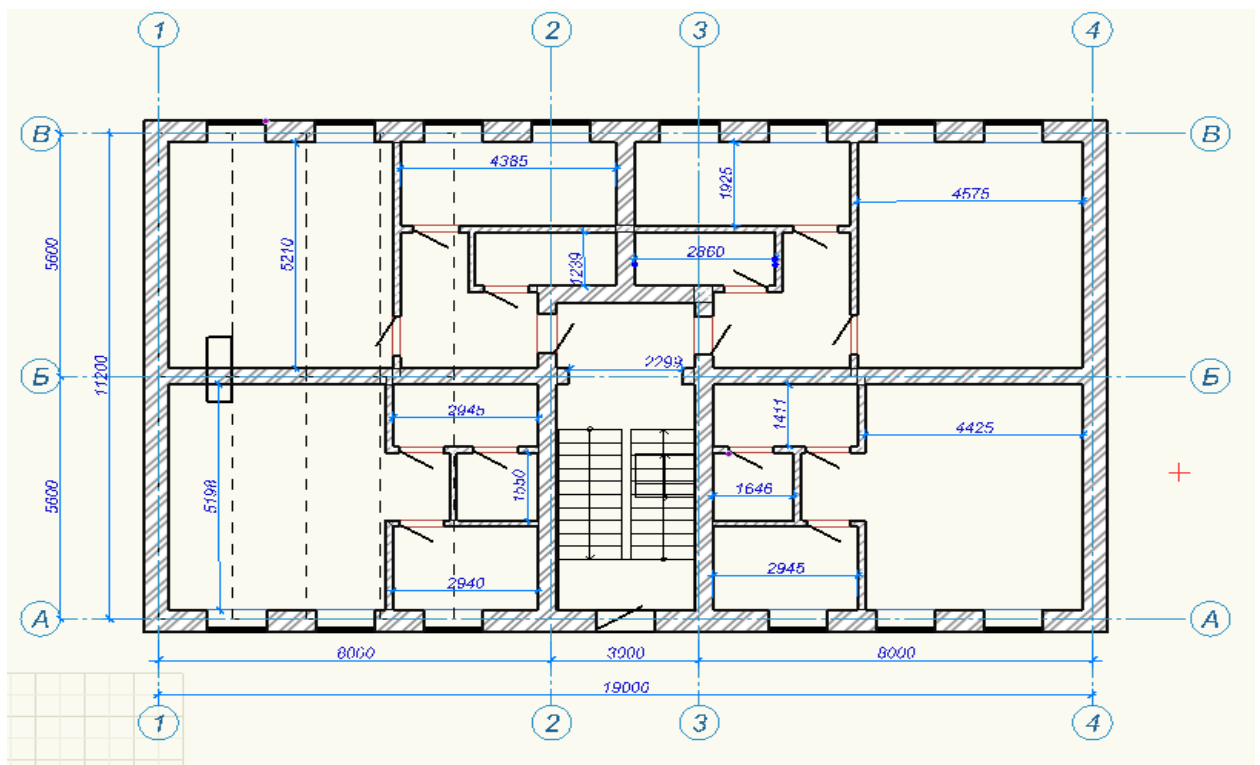
Рисунок 3. План первого этажа, полученный в ПК САПФИР
