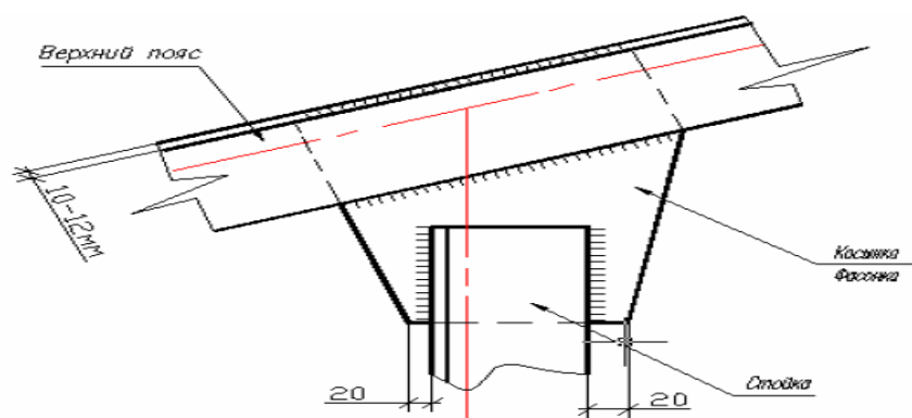
Рисунок 4. Элементы узла верхнего пояса фермы, их соединение сваркой
