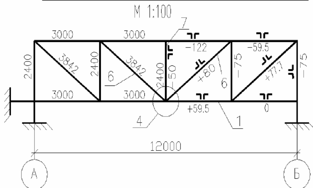
Рисунок 3. Геометрическая схема фермы
