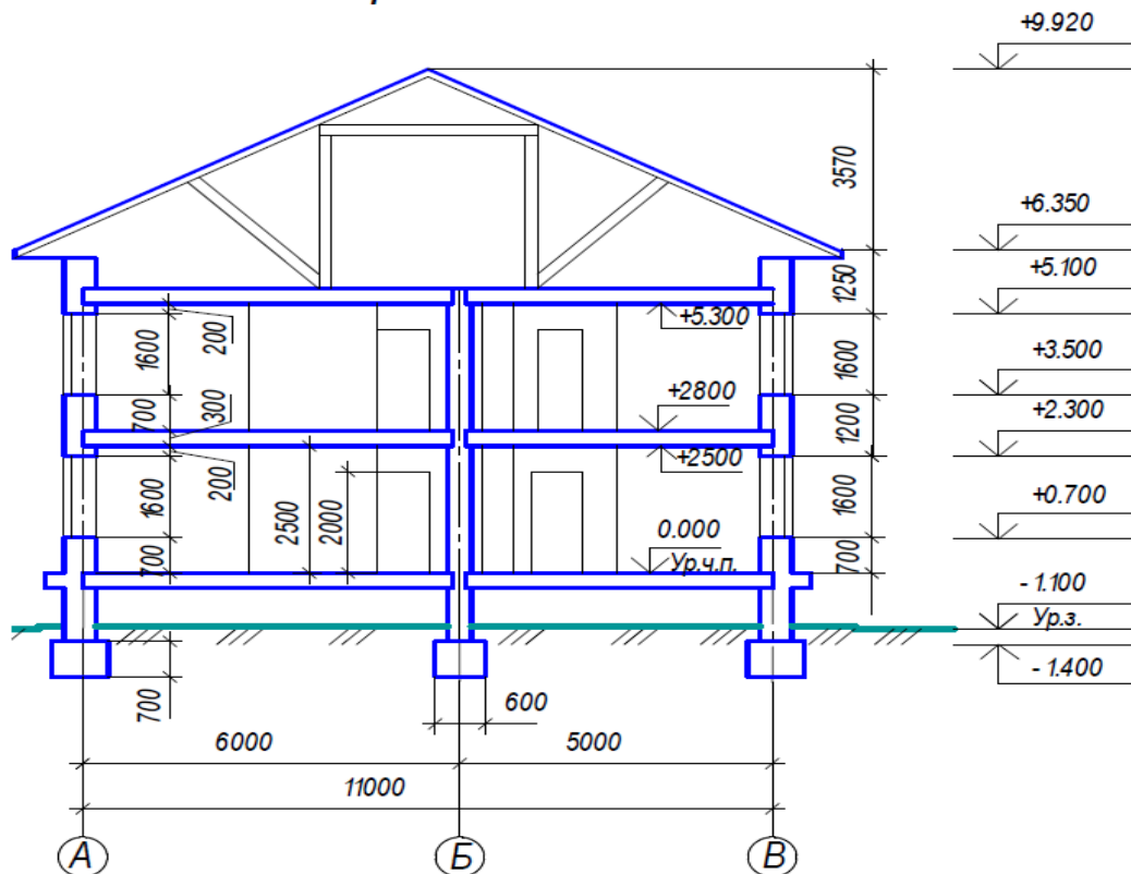
Рисунок 6. Разрез здания
