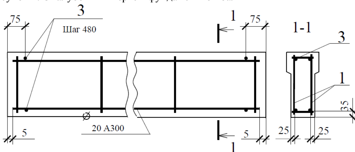
Рисунок 2. Схема армирования фундаментной балки
