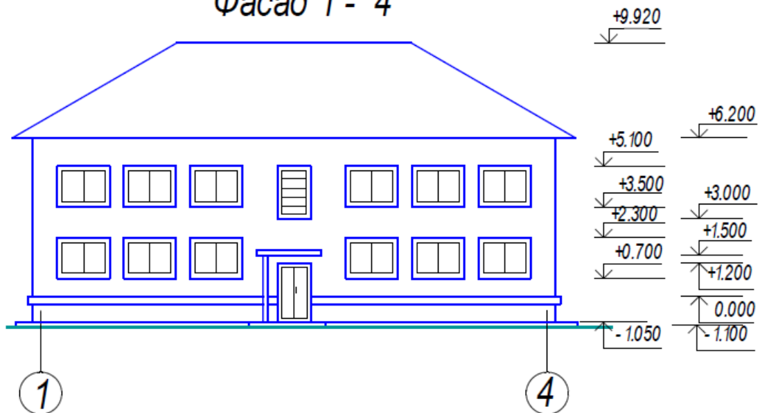
Рисунок 7. Фасад здания
