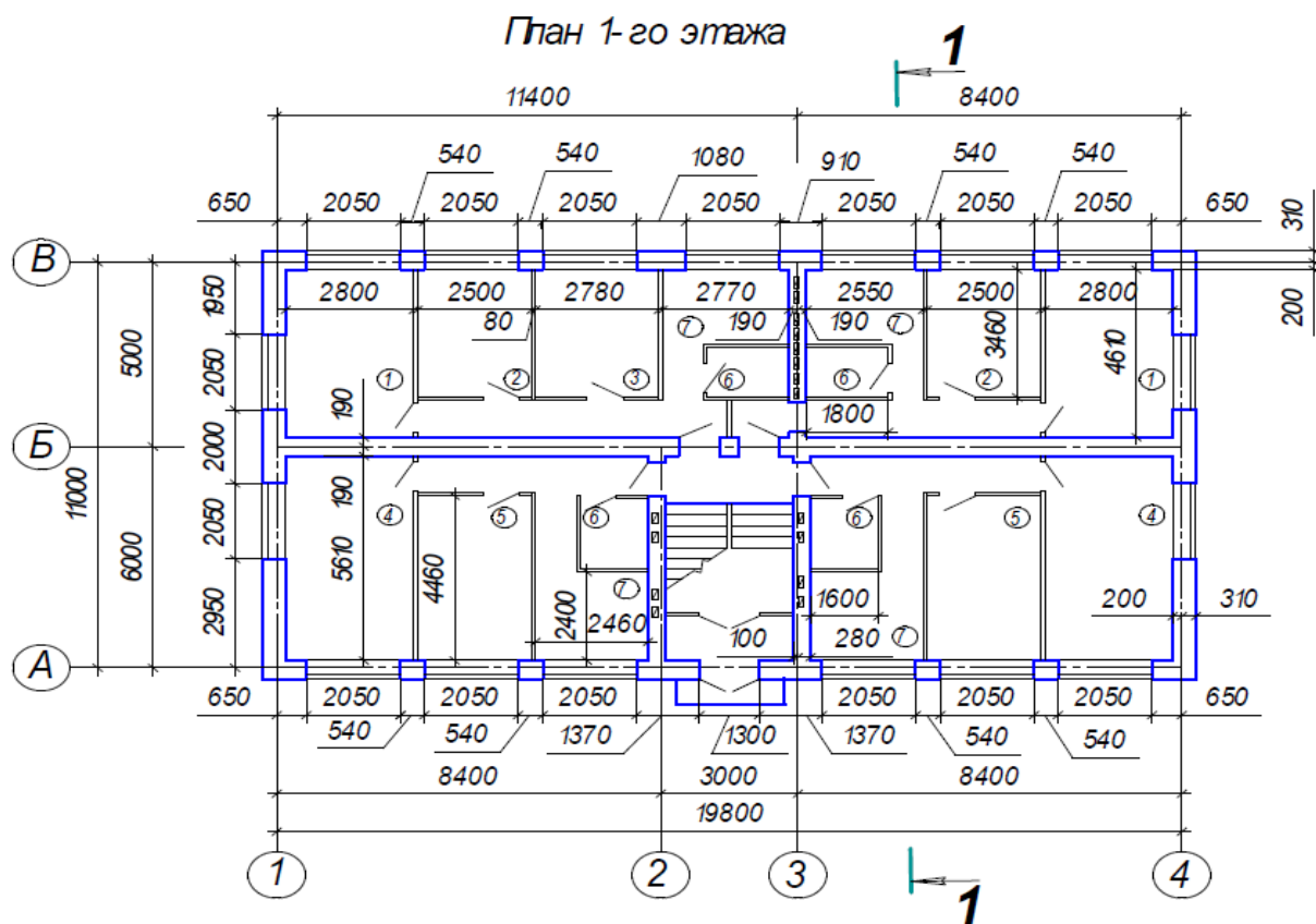
Рисунок 5. План первого этажа здания
