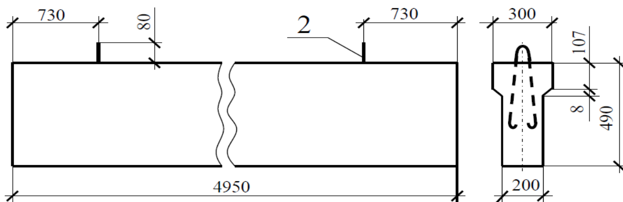
Рисунок 1. Опалубочный чертеж фундаментной балки
