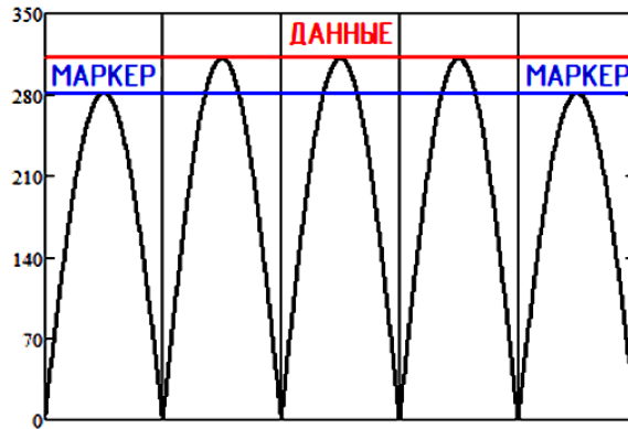
Рисунок 2 - Принцип модуляции данных в сети 220 В
