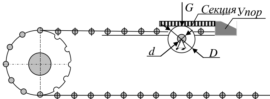
Рисунок 1- Схема перемещения секции тяговой секции
