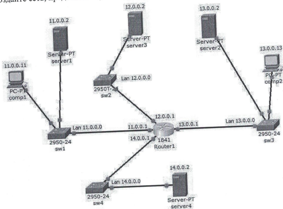
Рис. Схема корпоративной сети.
