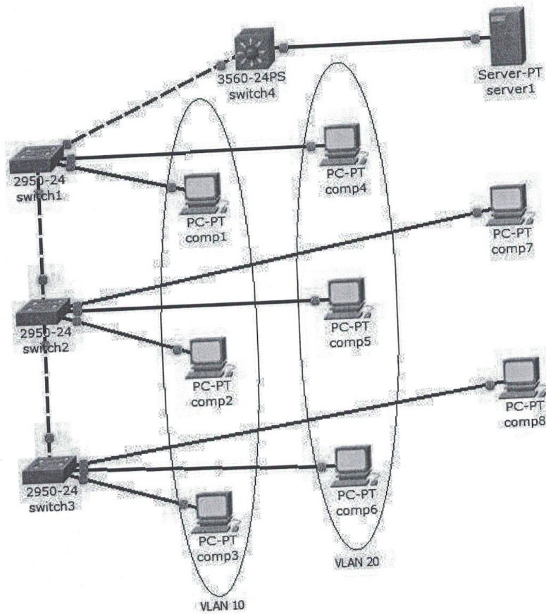
Рис. Схема корпоративной сети.
