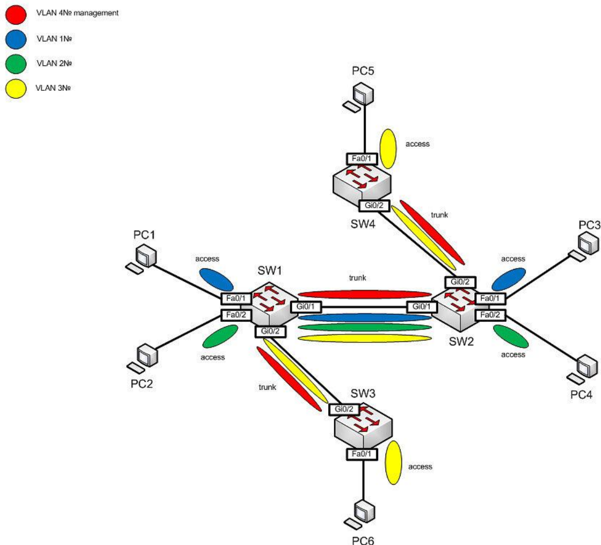
Рисунок Дизайн Vlan
