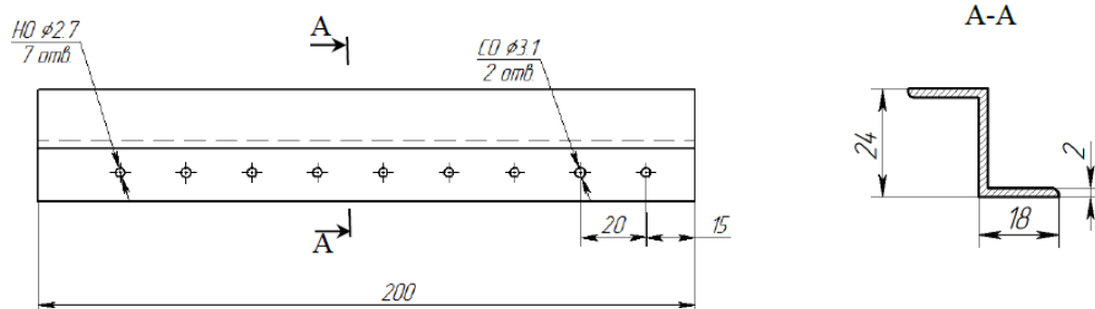
Рисунок 1 - Эскиз профиля зетового сечения
