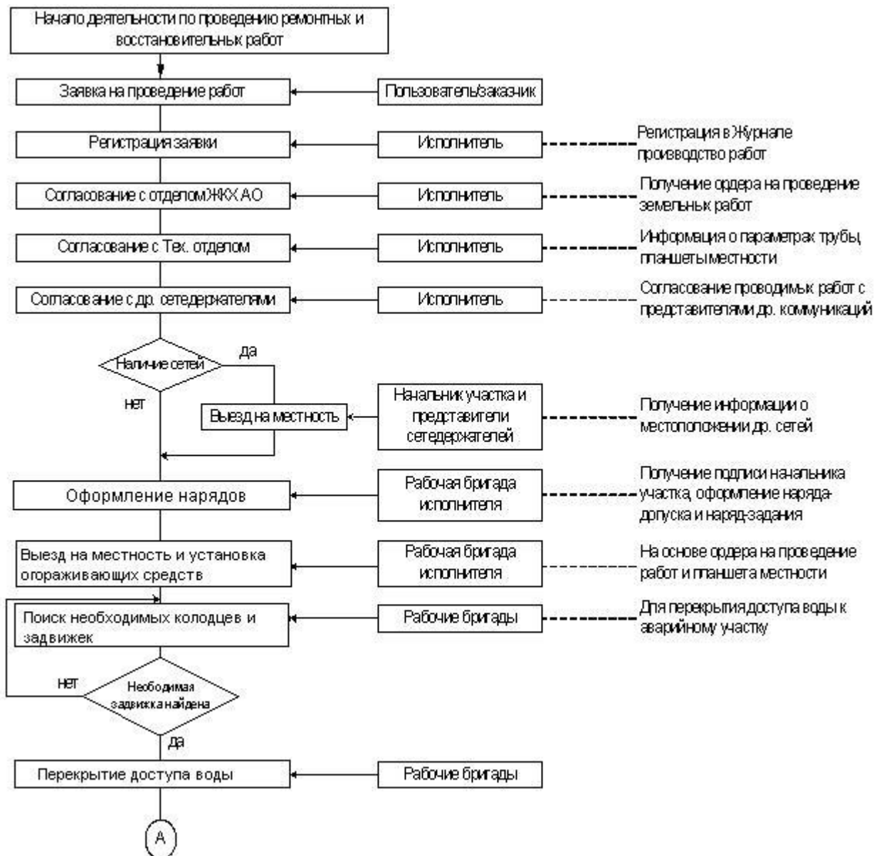
Рисунок 1 – Пример расширенной блок-схемы
