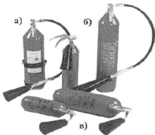
Рисунок А.1 – Общий вид углекислотных переносных огнетушителей
