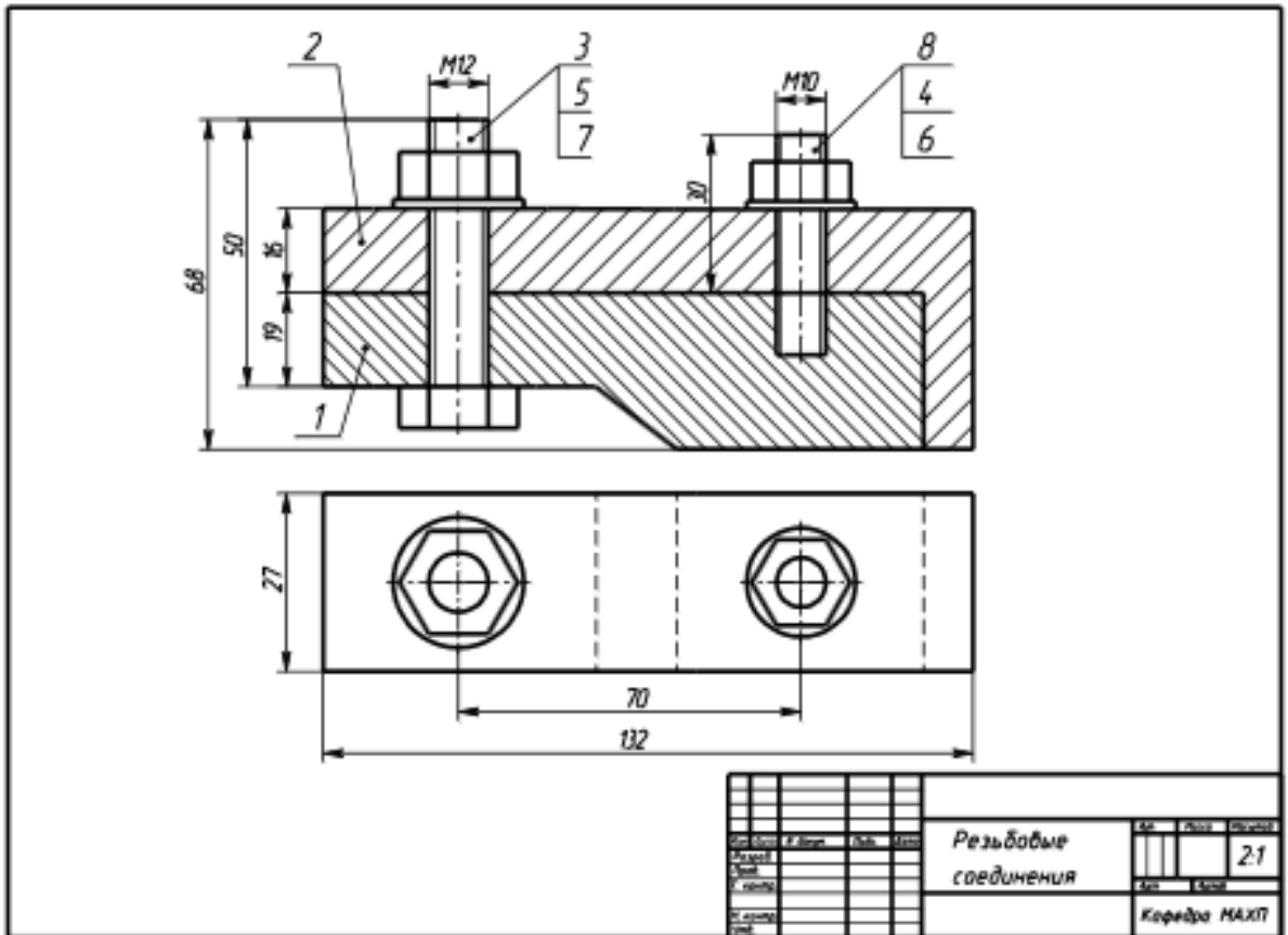
Рисунок 6. Вариант задания по резьбовым соединениям
