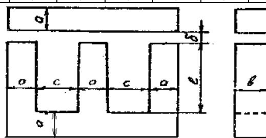
Рисунок 2 – Электромагнит с Ш-образным якорем
