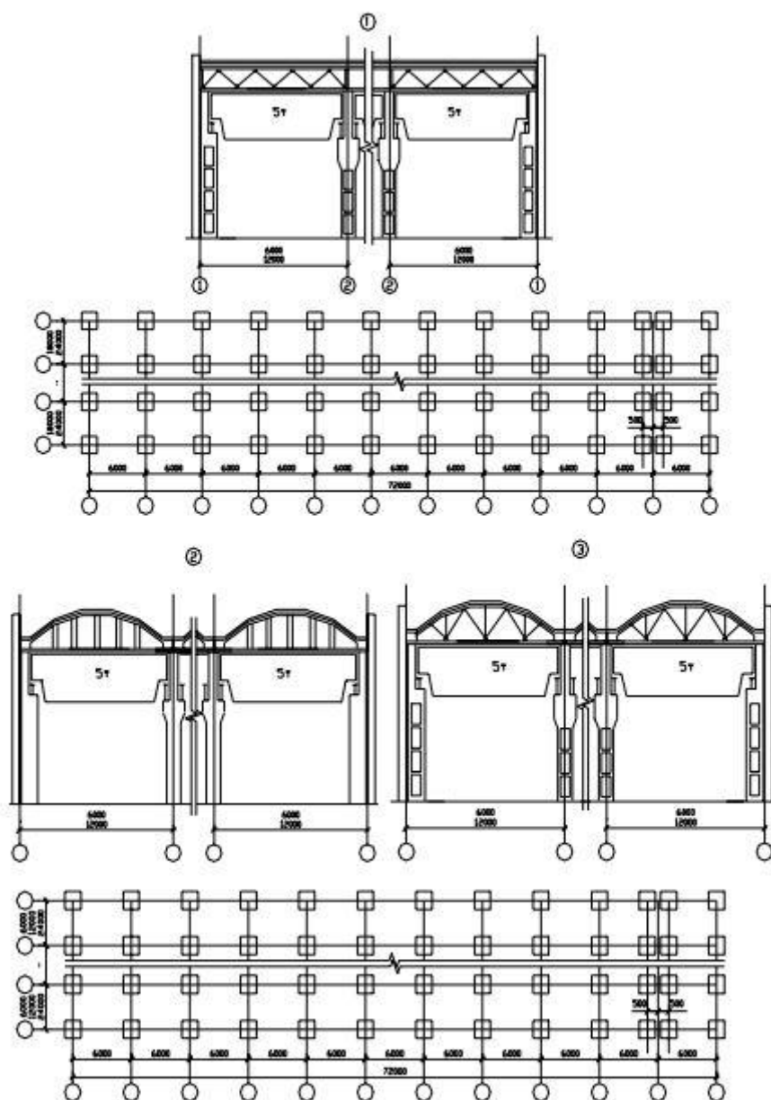
Рисунок 1. Схема зданий
