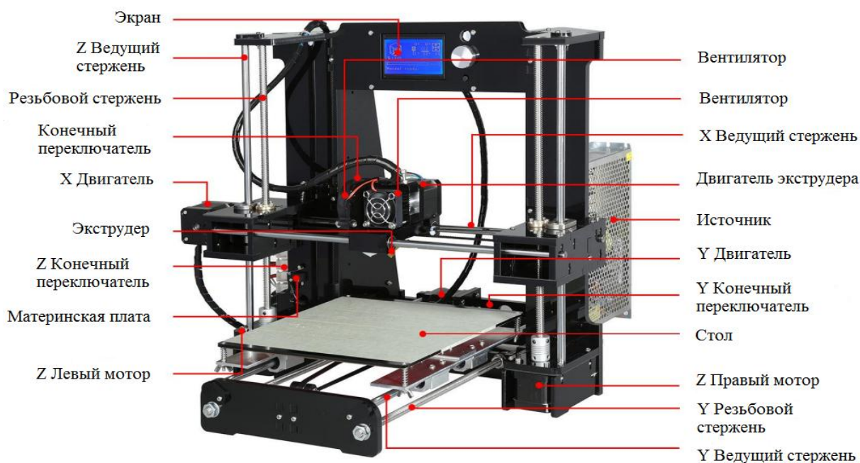
Рисунок 3.1- 3D принтер модели A6
