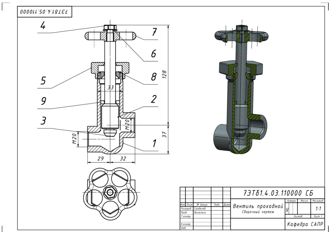
Рисунок 10 - Пример оформления сборочного чертежа для задания 4
