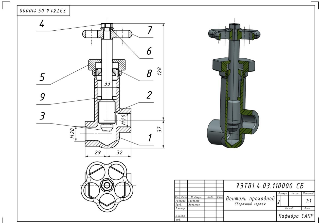
Рисунок 10 - Пример оформления сборочного чертежа для задания 3
