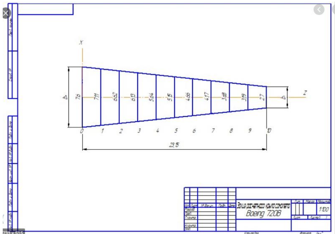
Рисунок 8 Профиль крыла самолета Voeng 720B
