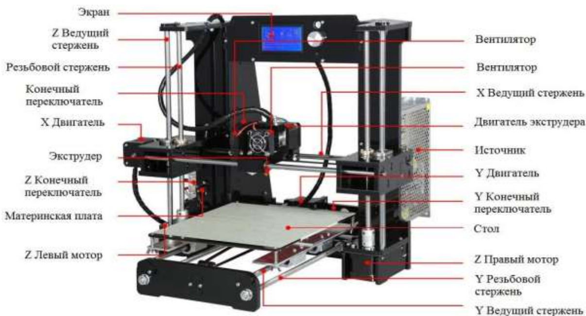
Рисунок 3.1- 3D принтер модели А6
